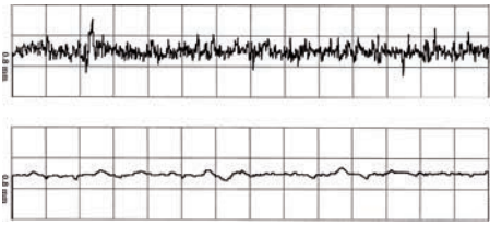
Profildigramme einer mit Korn 400 geschliffenen (oben) und einer mit Korn 120 und anschließend elektropolierten (unten) Edelstahloberfläche
